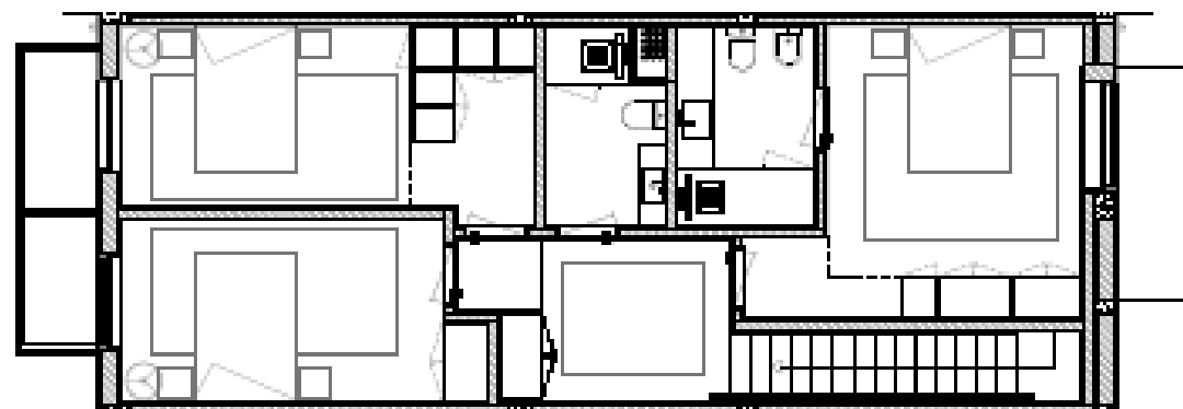
1º Piso
